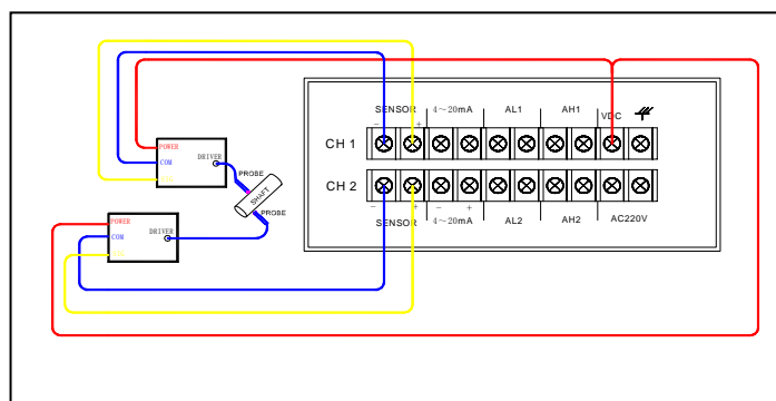
现场接线图
