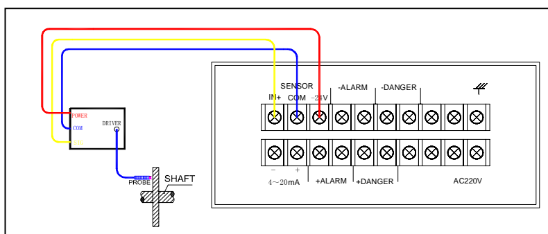
现场接线图
